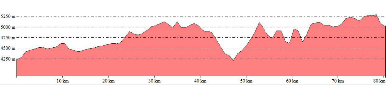
图 3 冈底斯成矿带深地震反射东剖面 II 段高程
