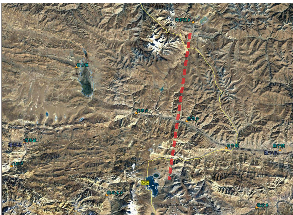
图 1 冈底斯成矿带深地震反射东剖面 II 段行政位置示意图
