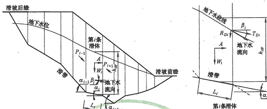
图 E.2 堆积层滑坡计算模型之二:传递系数法(折线型滑动面)
