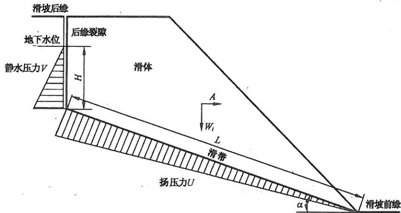
图 E.3 岩质滑坡计算模型:极限平衡法
