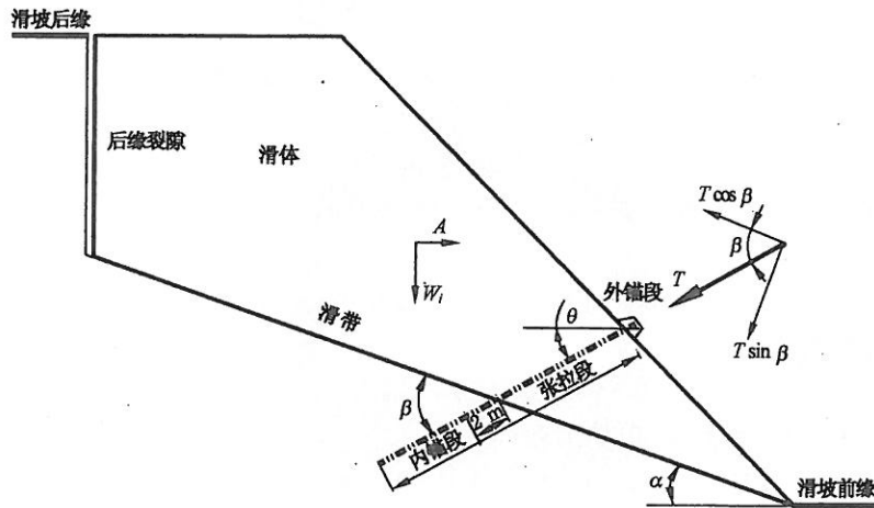
图 E.4 预应力锚索对滑坡作用示意图
