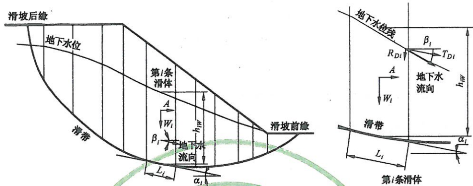
图 E.1 堆积层滑坡计算模型之一：瑞典条分法(圆弧型滑动面)
