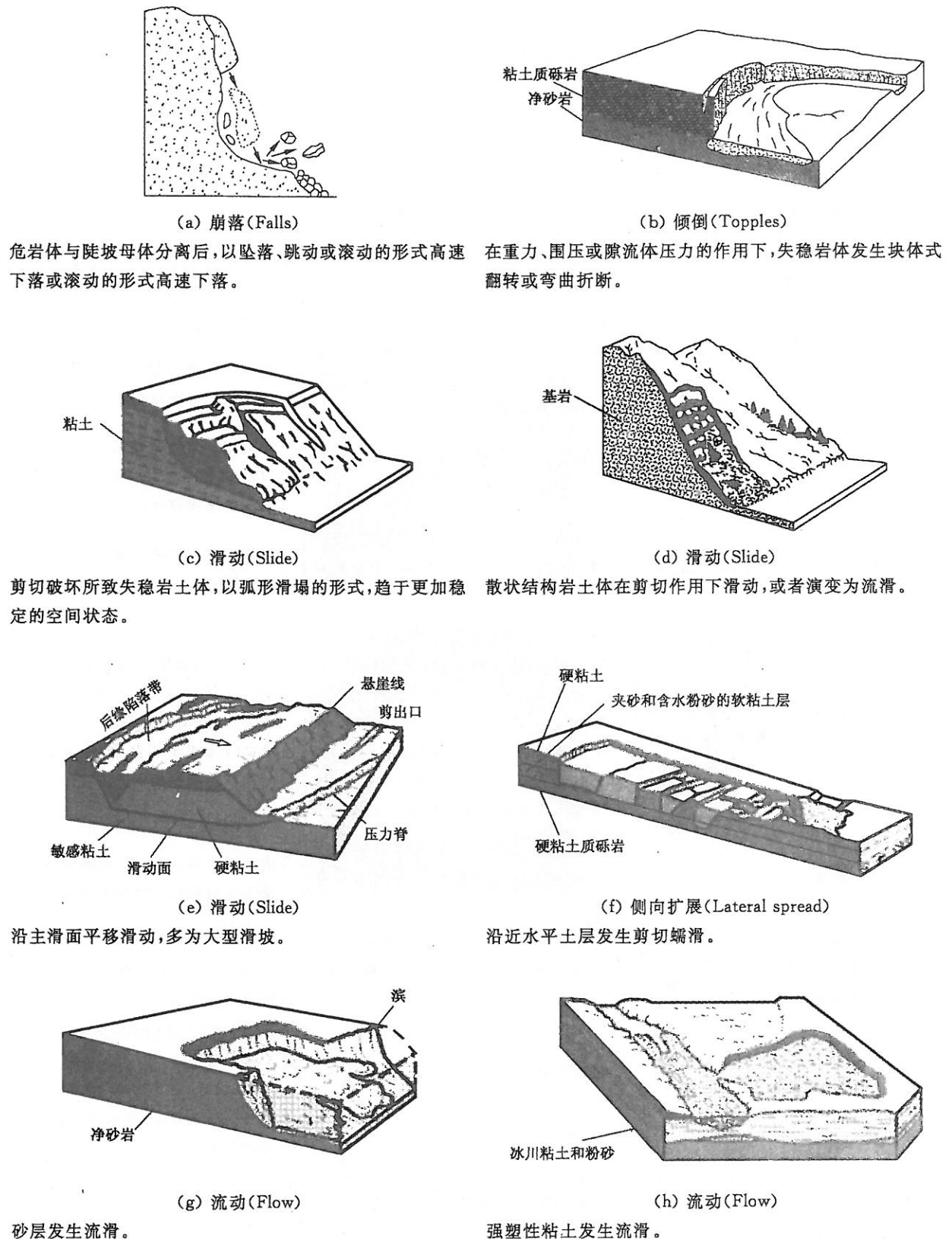
图 A.2 典型滑坡实例示意图(依据瓦恩斯,1978)
