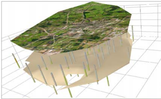
上海青浦新城第二硬土层三维结构
