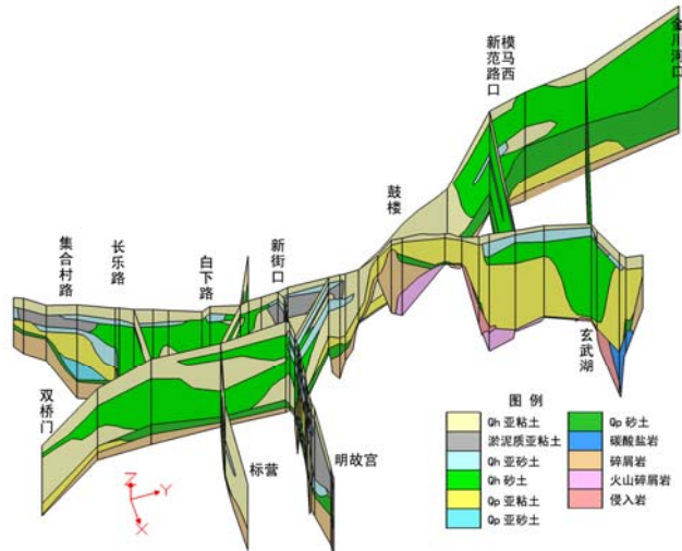
南京市区长江分支河道孔隙含水层组三维结构
