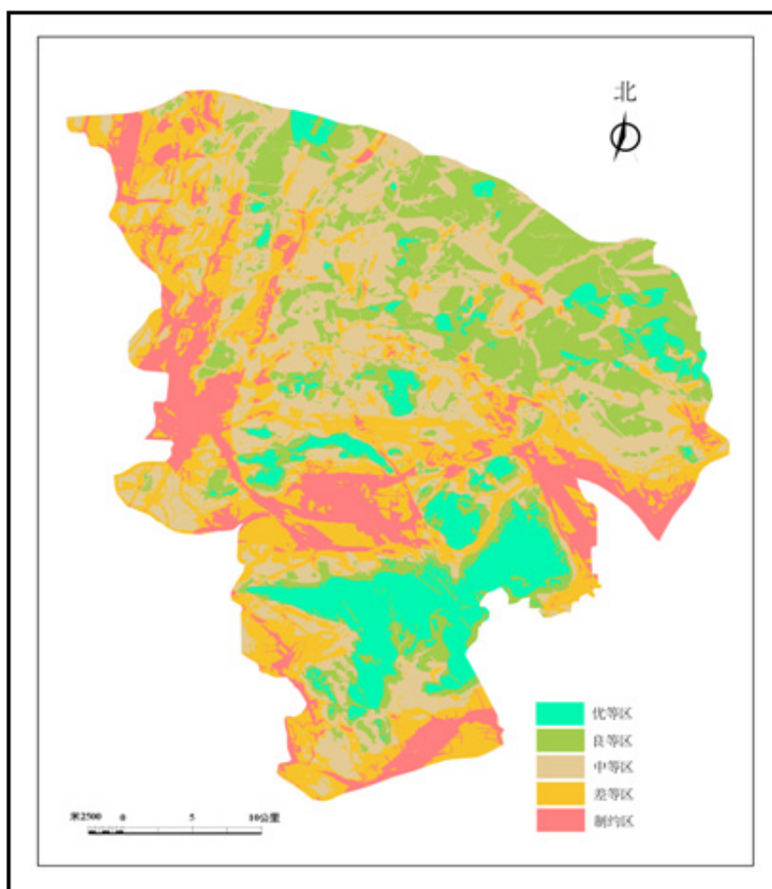
广州中心城区—番禺区浅层地下空间资源质量综合评价图
