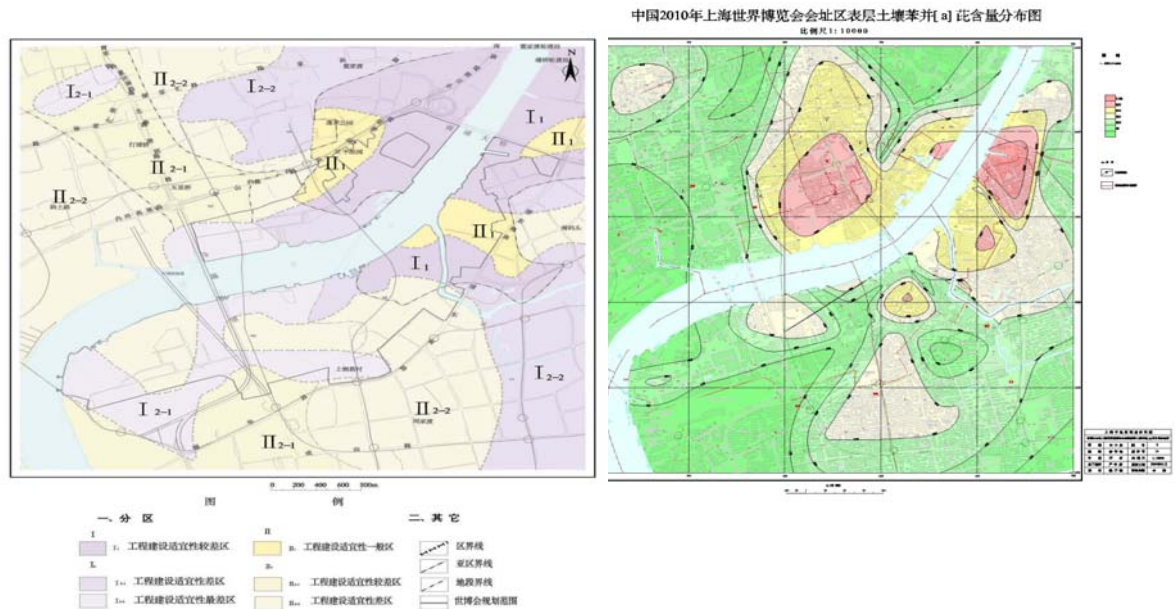
世博会址区基坑工程建设适宜分区
