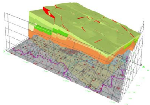
天津三维基岩地质结构模型
