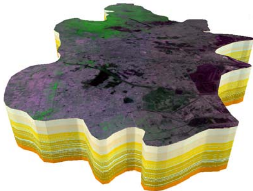
天津平原区水文地质三维地质结构
