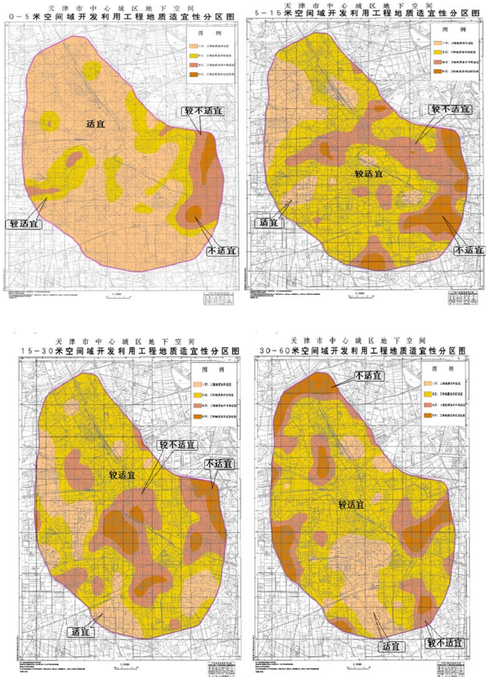
天津市中心城区地下空间开发利用工程地质适宜性分区图
