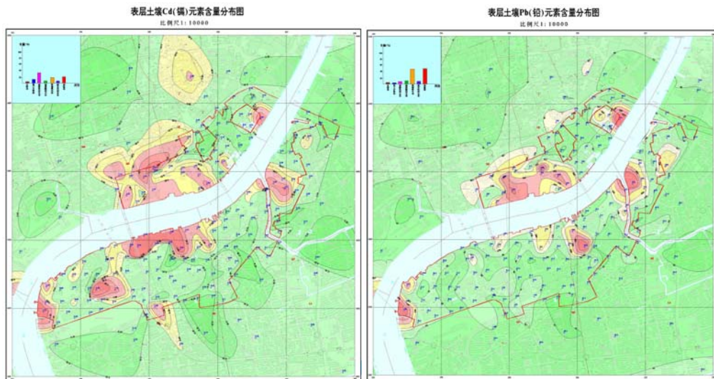
世博会址区表层土壤镉、铅分布图
