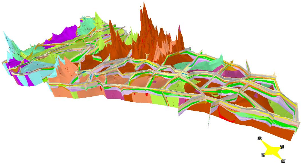
广州南沙片区第四纪松散沉积层三维地质结构
