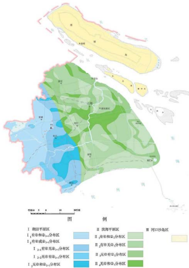
上海市工程地质结构分区图
