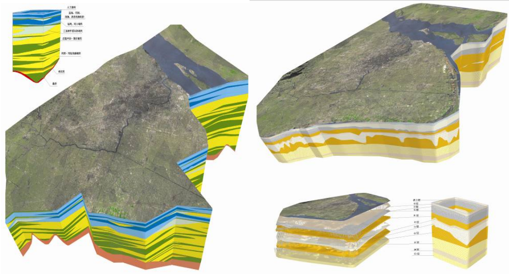
上海市第四系地质结构和100M以浅工程地质结构模型图
