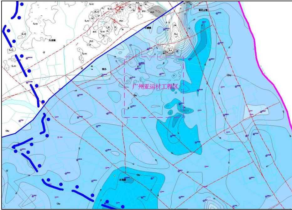
广州市亚运村工程断裂构造图
