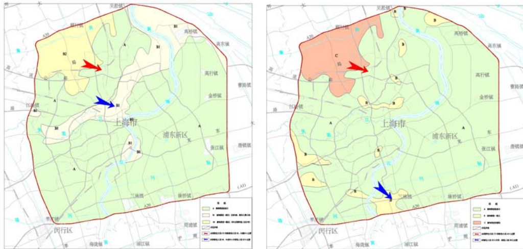
上海中心城区 20-25 米、10-20 米隧道盾构考虑掘进面土层变化情况推进 适宜性分区
