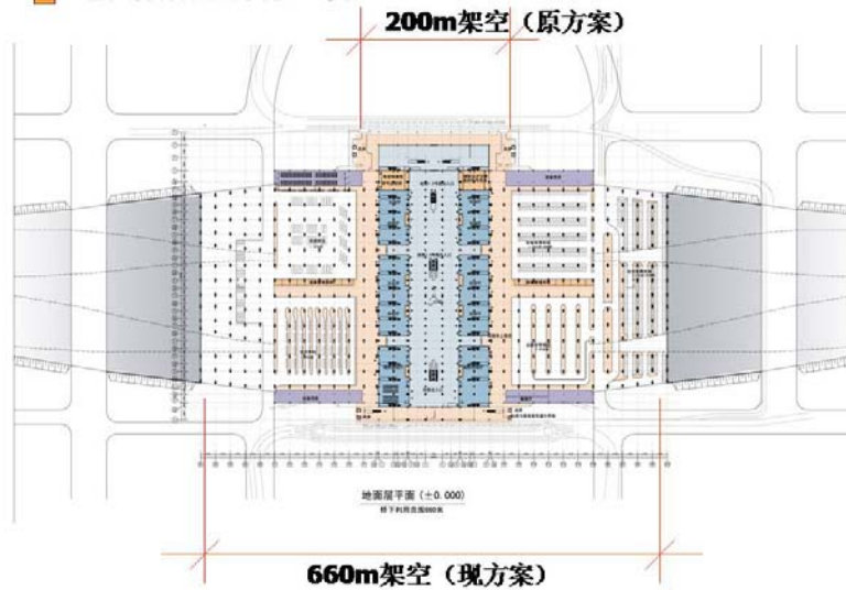
南京火车南站地面层架空方案比较
