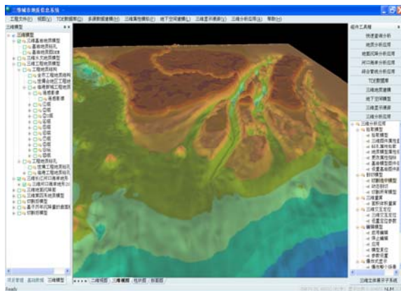
上海河口海岸演化模型
