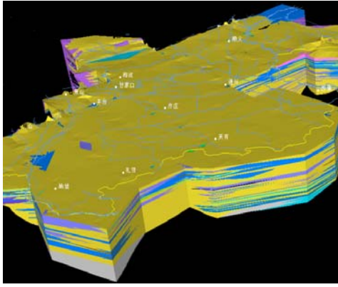
北京市平原区基岩和第四系三维地质结构
