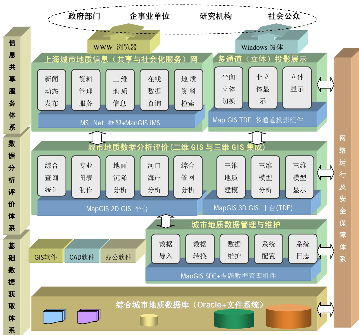
系统软件体系结构
