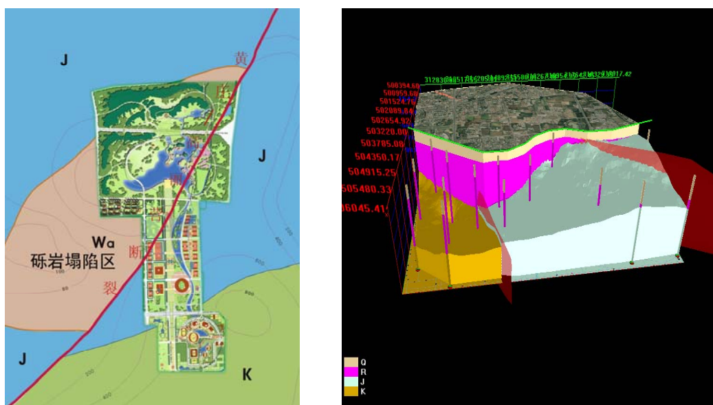
北京奥运场馆区隐伏岩溶塌陷区、活动断裂分布图
