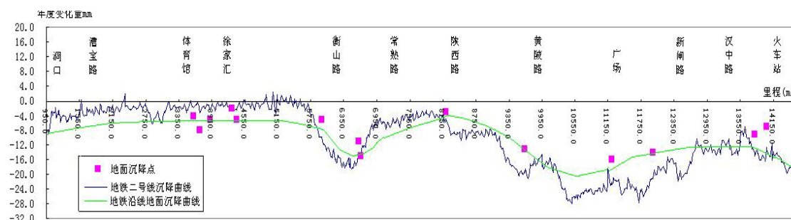
上海地铁二号线地面沉降监测曲线图
