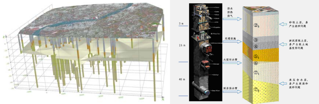
世博会会址区地下三维结构
