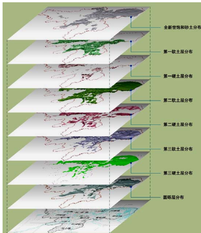
杭州市三维工程地质结构特征
