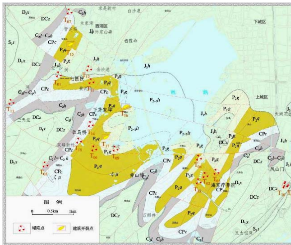
杭州西湖地区岩溶塌陷分布
