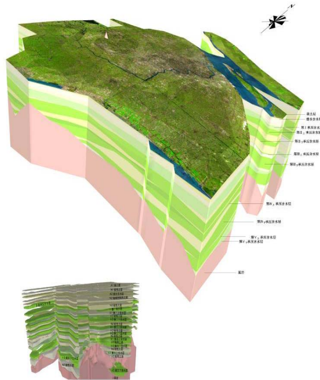
上海市三维水文地质结构图
