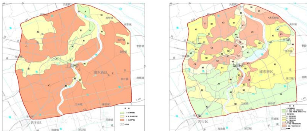
上海中心城区 20 米基坑软土变形、30 米基坑考虑流砂问题适宜性分区
