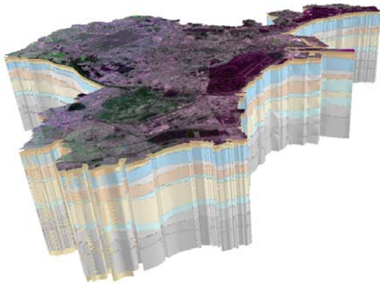
天津中心市三维工程地质地质结构
