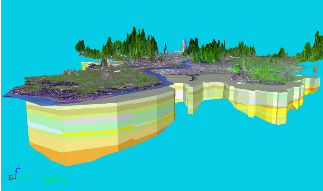
杭州市三维第四纪地质结构
